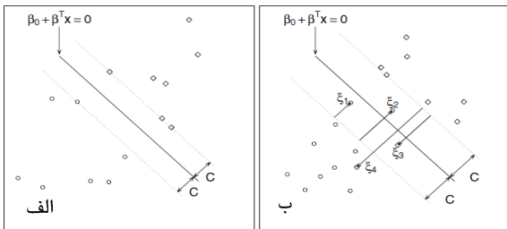
شکل ۱. مدل‌های رده‌بندی ماشین بردار پشتیبان خطی الف: حالت غیر قابل جداسازی ب: حالت قابل جداسازی [۲۰]
